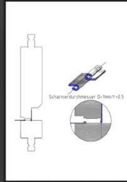
Scharnierwerkzeug hinge tool
