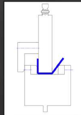
U-Bieger mit unterschiedlichen Winkeln U-bend with different angles
