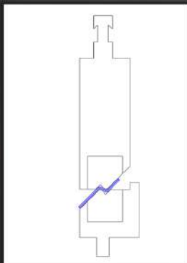
Z-Bieger auch als Halter+Einsatz Z-bending tool
