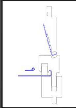
Einroll-Scharnierwerkzeug (2x Hub) enroll-hinge tool, 2 hubs
