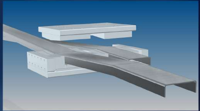
Biegewerkzeug U-Profil Bending tool U-profile
