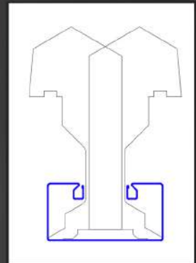
OW Schwenkbiegewerkzeug pan-bending tool
