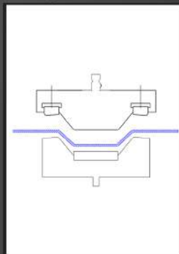
Trapezwerkzeug, Winkel und Profiltiefe einstellbar trapezoid tool
