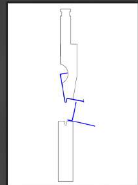
Präge + Zudrückwerkzeug stamp + press tool
