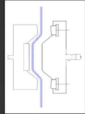
Trapezwerkzeug mit verstellbaren Leisten trapezoid tool with movable bars
