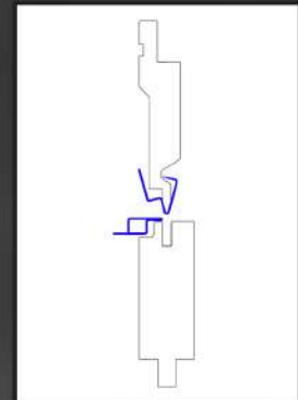
Falz- und Zudrückwerkzeug (geschlossenes Profil) fold + press tool
