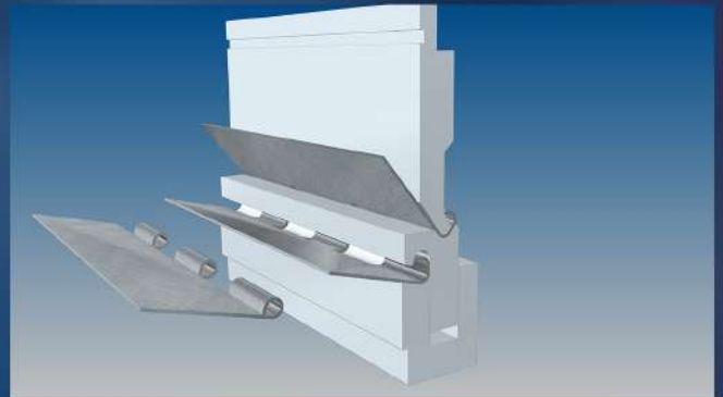
Scharnier-Werkzeug (3 Hübe)
