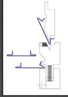
Präge + Falzwerkzeug stamp + fold tool
