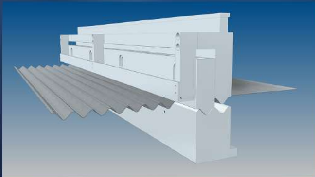
Wellblech-Werkzeug
