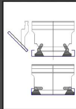
Klapphörner (Rahmenprofil) flap-horn tool
