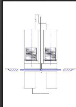
Prägewerkzeug mit Niederhalter (Kalotte Rund stirnseitig) stamp tool with holder
