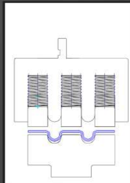
Prägewerkzeug Hutprofil Rund mit Niederhalter stamp tool (hat profile)
