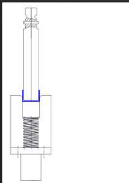
U-Bieger mit Auswerfer U-bend with ejector
