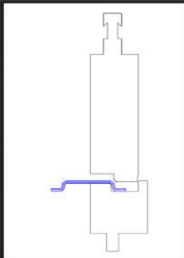
Absetzwerkzeug spreading tool
