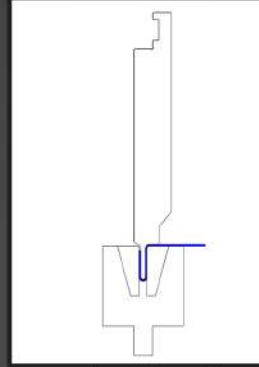
Prägewerkzeug Hutprofil einseitig stamp tool (hat profile, single sided)
