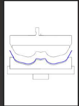
Prägewerkzeug stamp tool
