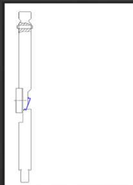
Z-Bieger Werkzeug mit Anschlag Z-bending tool with stop bar
