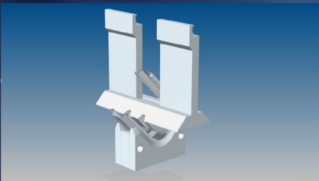
Umformwerkzeug Blechprofil reshaping tool metal profile
