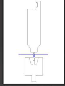
Prägewerkzeug Hutprofil beidseitig stamp tool (hat profile, double sided)
