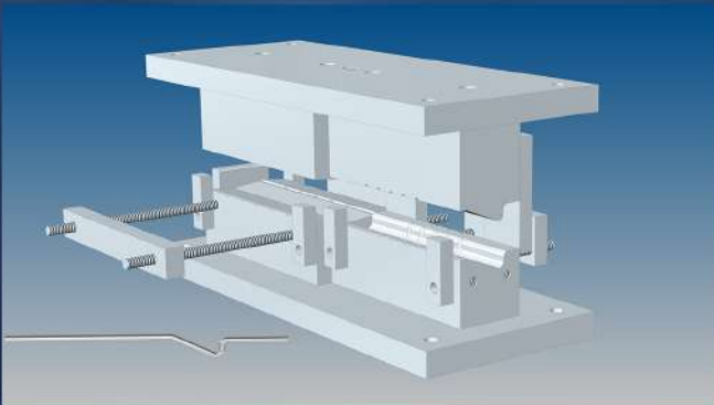
Mehrfach-Stationenwerkzeug für Draht Multi-station tool for wires
