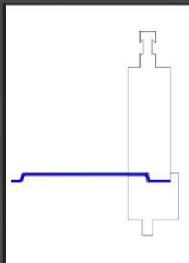
Absetzwerkzeug mit Querverriegelung spreading tool with cross block
