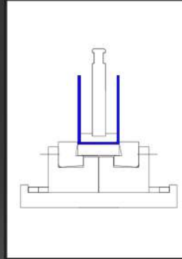
U-Bieger 2x90°, Öffnungsweite verstellbar U-bending tool
