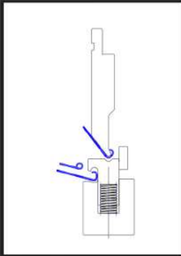
Einroll-Scharnierwerkzeug (3x Hub) enroll-hinge tool
