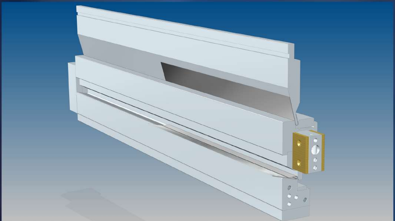
Etagenwerkzeug für geschlossenes Profil
