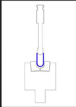
U-Bieger Radius mit Schwenkbacken U-Bend radius with pan-shoe
