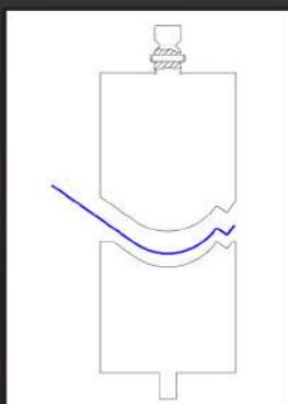
Prägewerkzeug Radius + Z-Kantung stamping and radius tool
