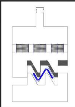
Absetzwerkzeug mit Niederhalter für Z-Profil spreading tool with holder
