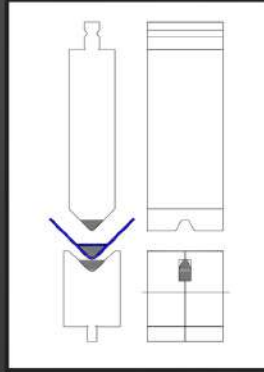
Quersickwerkzeug (Versteifungssicke) cross-bead tool
