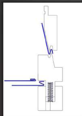
Präge-Falzwerkzeug (Doppelfalz) stamp-fold tool
