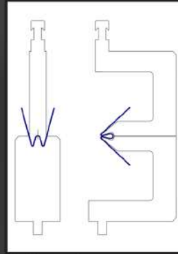
Stationswerkzeug geschlossenes Profil station tool (closed profile)
