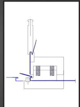
Etagen-Zargenwerkzeug floor-rib tool
