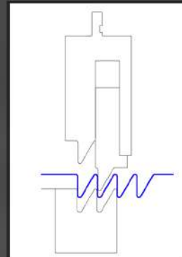
Wellblechwerkzeug mit Niederhalter corrugated iron tool with holder
