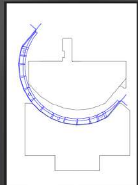
Prägewerkzeug Steppprofil + stirnseitige Aufkantung stamping tool,
