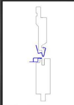
Falz + Zudrückwerkzeug (geschlossenes Profil) fold + press tool
